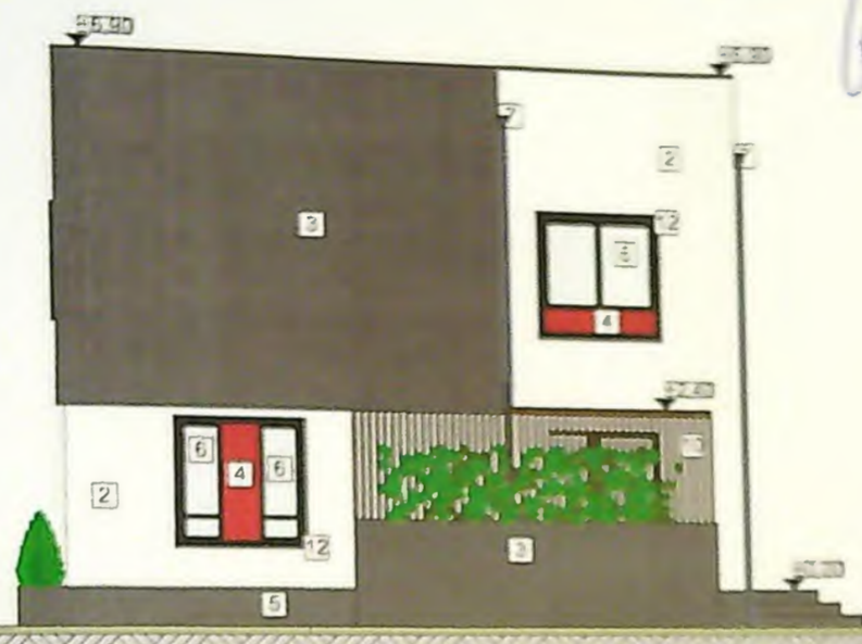
Fațadă lateral dreapta -vest scara 1:100
