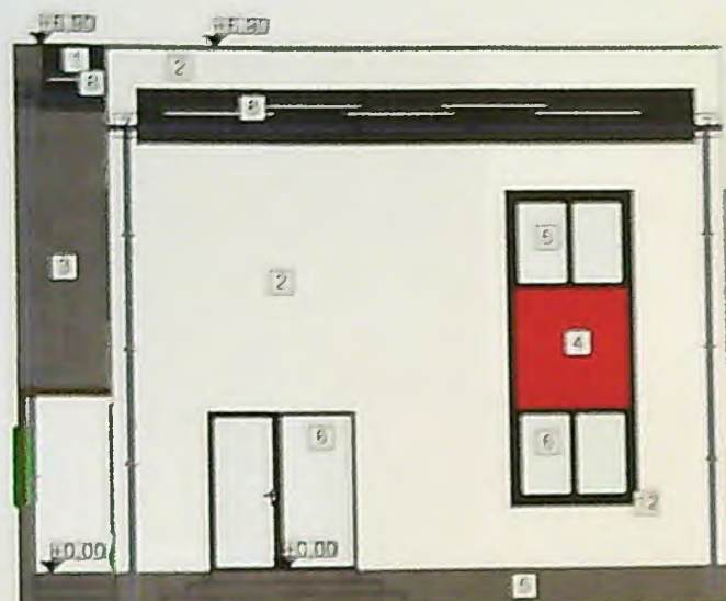
Fațadă posterioară locuință -Sud scara 1:100
