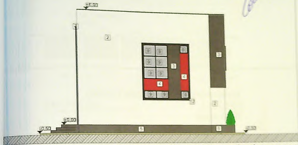
Fațadă lateral stânga -est scara 1:100
