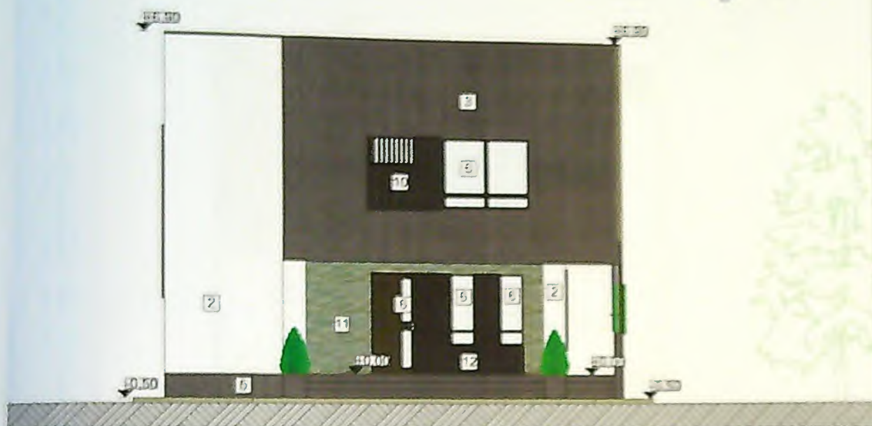
Fațadă principală locuință - Nord scara 1:100
